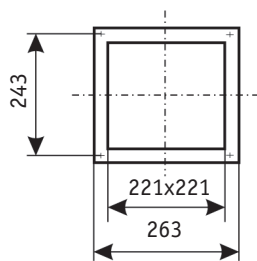
Выходной фланец
